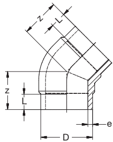
25.15.01.101 PE100 Winkel 45° kurz SDR11 schwarz PE100 Elbow 45° short SDR11 black
